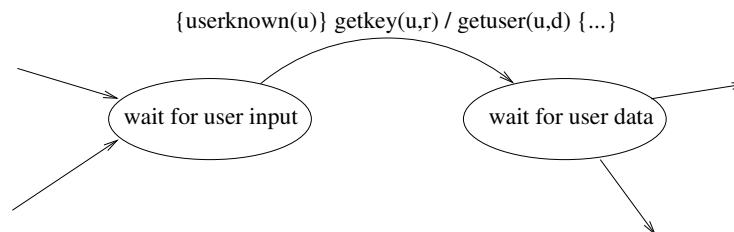
Abbildung 5.6: Zustandsautomat
