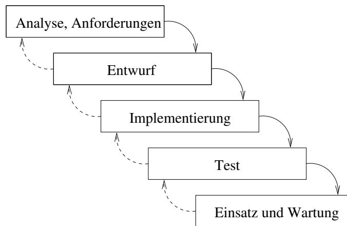
Abbildung 2.1: Wasserfallmodell
