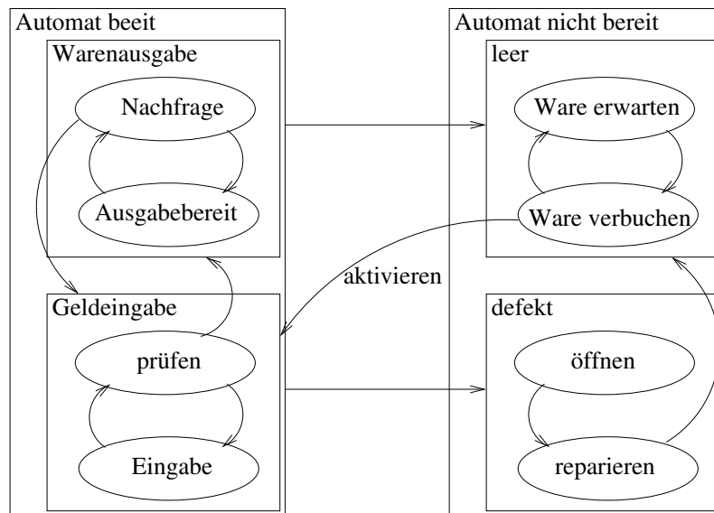
Abbildung 3.9: Statechart
