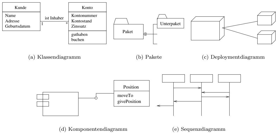
Abbildung 3.10: UML – Diagramme
