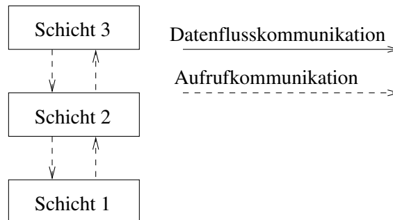
Abbildung 5.2: 3 – Schichten – Architektur
