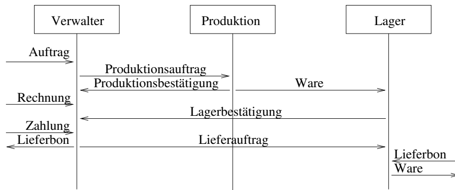
Abbildung 3.5: Interaktionsdiagramm
