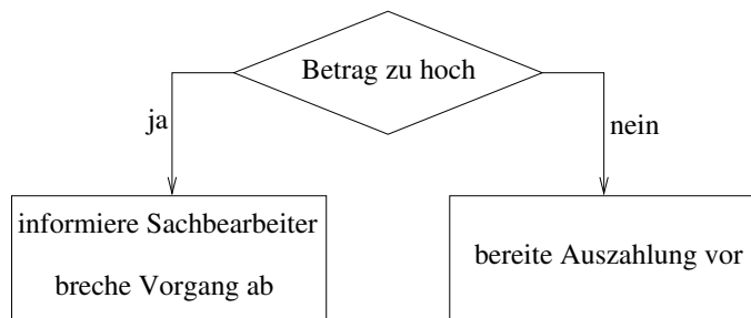
Abbildung 3.1: Kontrollflussdiagramm
